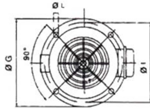
Pompe machine-outil triphasée 220/380V
